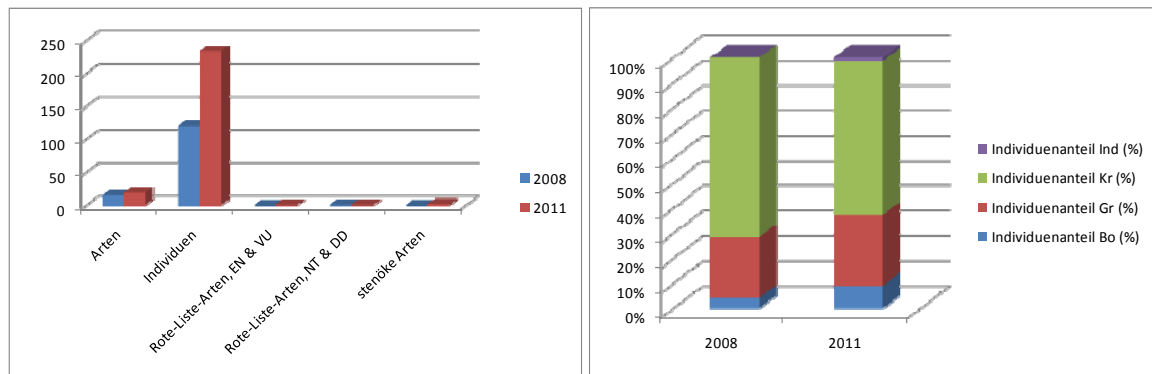
Abbildung 105 und Abbildung 106: Flächen 15, Vergleich 2008 und 2011. Wanzenarten- und -individuenanzahl sowie Anzahl von Rote-Liste-Arten und von stenöken Arten (links) sowie Individuenanteile unterschiedlicher ökologischer Gilden, gestapelt (rechts). EN = stark gefährdet, VU = gefährdet, NT = nahezu gefährdet, DD = Datenlage ungenügend; Bo = Bodenbewohner, Gr = Grasbesiedler, Kr = Kräuterbesiedler, Ind = indifferente Arten.
